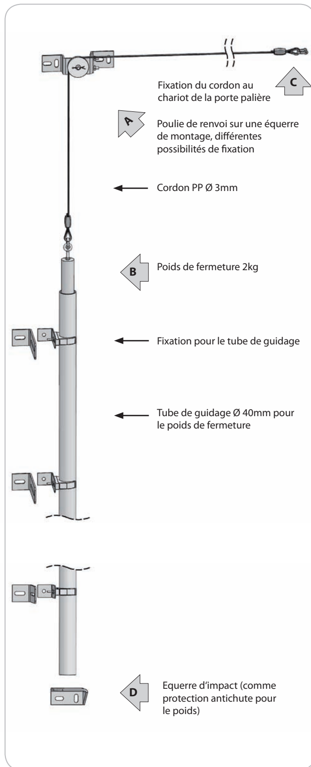
C Fixation du cordon au chariot de la porte palière
