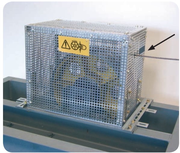
Exemple de montage sur un bâti de machine avec une sortie de câble horizontale.
